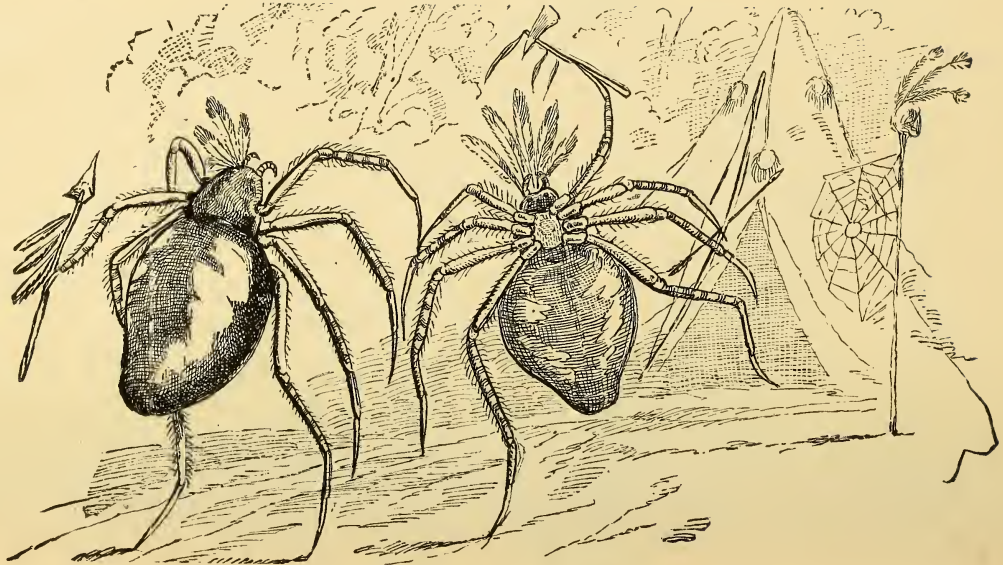
FIG. 7.—“SCALPAGE.”—(p. 34.)
